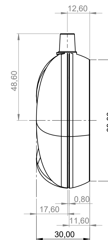
Seitenansicht links left lateral view
