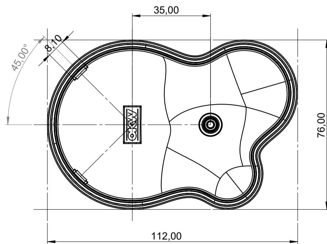
Unterteil - Innenansicht bottom part - inside view
