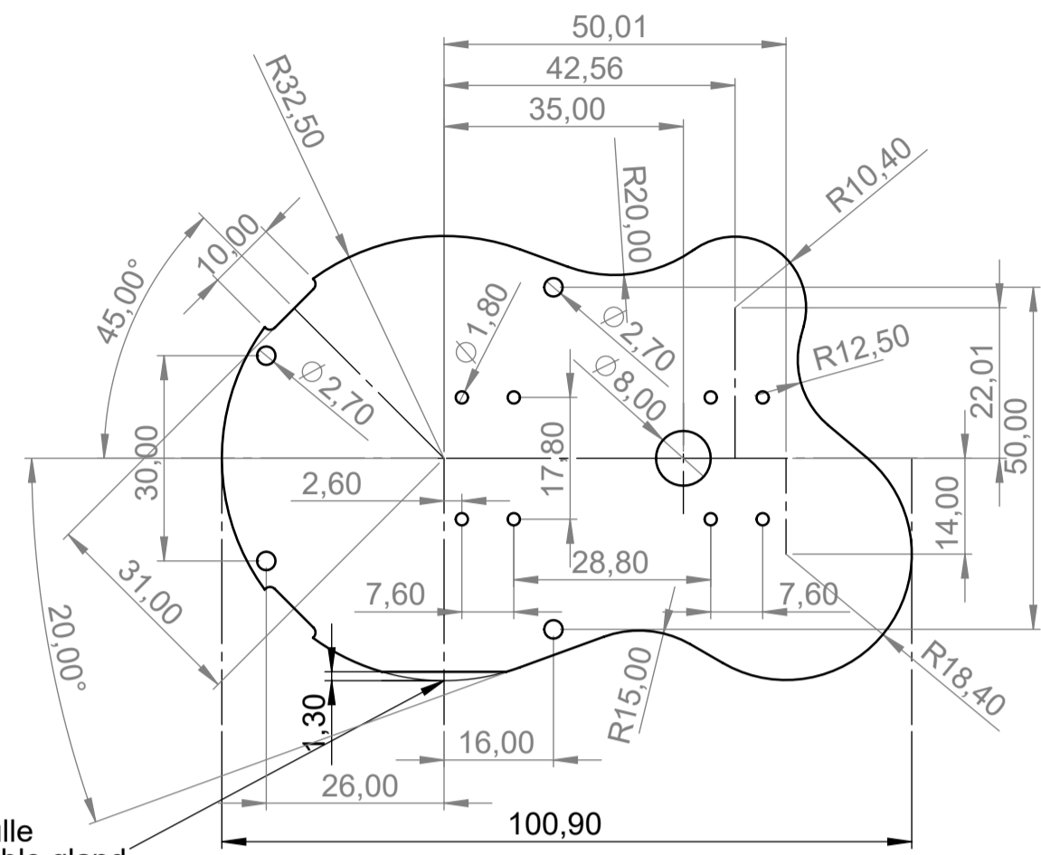
Beispielplatte mit platzierten Bohrungen für die AAA Kontaktclips sample PCB with placed holes for the AAA battery clips
