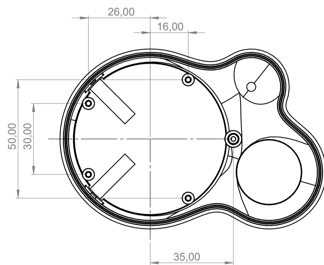
Oberteil - Innenansicht top part - inside view
